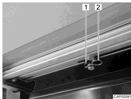
Fig. 73 Asta di azionamento (scalino di ingresso)
