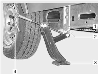
Afb. 172: Wagenkrik, AL-KO
