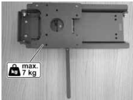
Afb. 65: TV-wandhouder, voorbeeld
