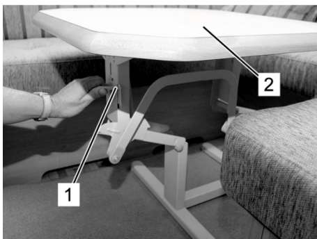
Afb. 138: tafel met heftafeldraagconstructie
