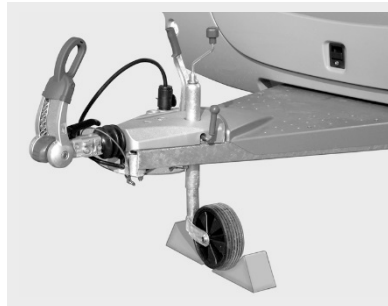
Afb. 169: Steunwiel borgen
