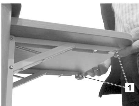
Afb. 145: Vergrendeling losmaken
