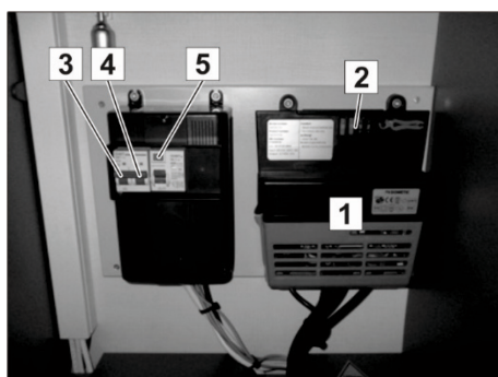
Afb. 67: Omvormer (netvoeding) (1) en zekeringautomaten
