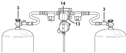
Afb. 110: Gasdrukregelset
