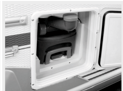
Fig. 50 : Cassette WC avec manchon de remplissage de la chasse d'eau
