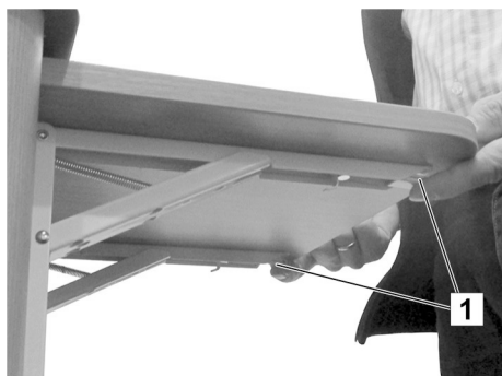
Fig. 208 : Défaire l'arrêt de la console pliante
