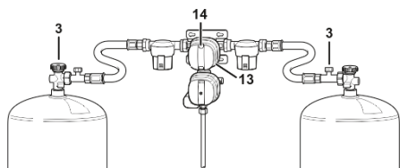
Fig. 117 : Kit détendeur
