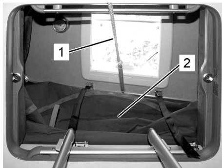
Fig. 194 Câble de traction (1), soufflet (2)
