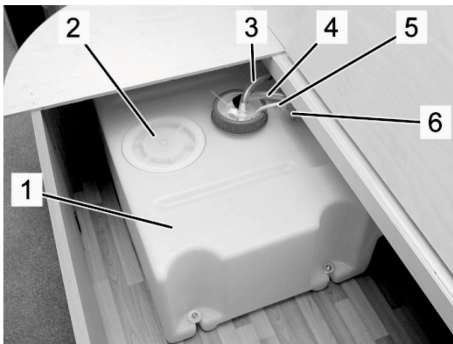
Fig. 96: Exemple de réservoir d'eau fraîche
