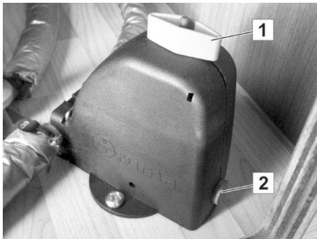
Fig. 111 : Vanne de vidange de sécurité ouverte
