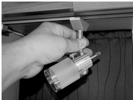
Fig. 191 : déplacer les spots LED
