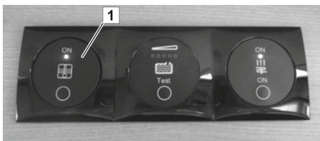
Fig. 102 : Boutons Marche/Arrêt pour la production d'eau chaude
