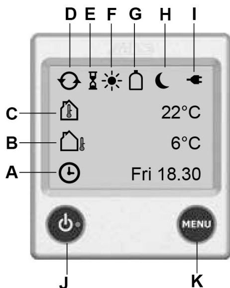
Fig. 88 : Éléments de commande
