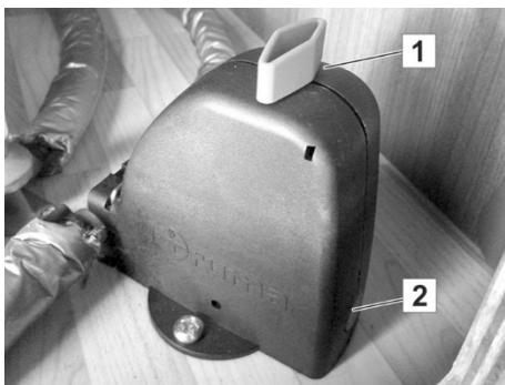
Fig. 112 : Vanne de vidange de sécurité fermée
