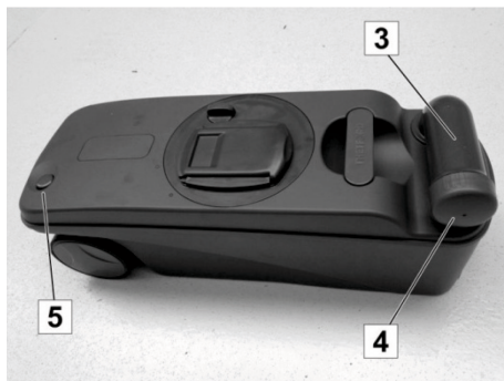
Fig. 200 : Vidange de la cassette WC
