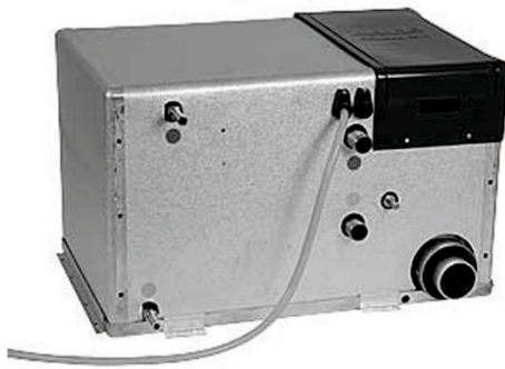
Fig. 87 : Chauffage ALDE
