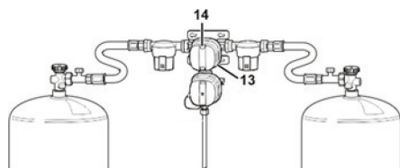
Fig. 120 : Kit détenteur
