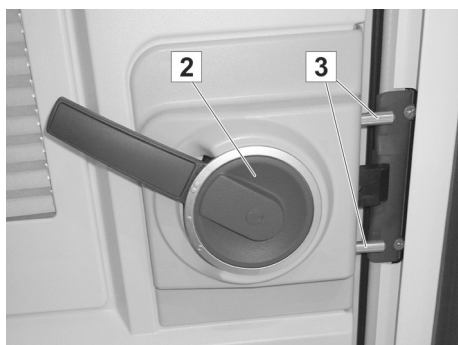
Fig. 17 : Porte fermée et sécurisée
